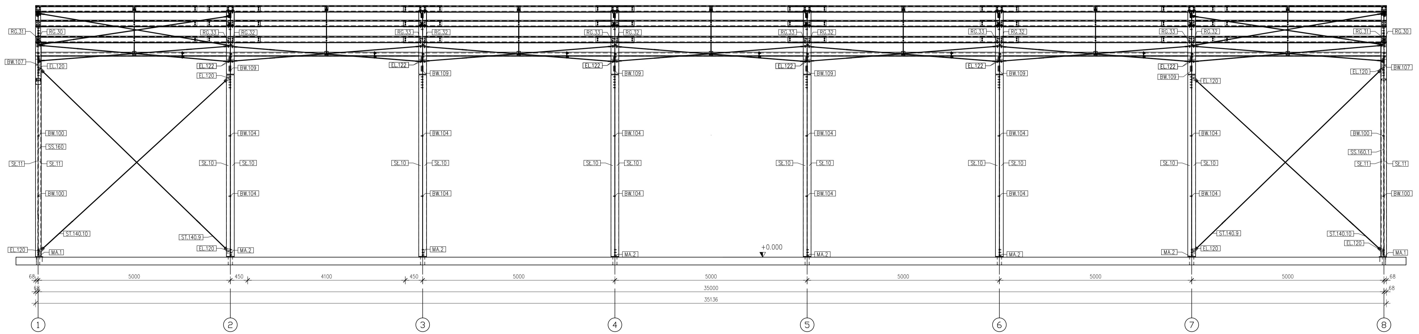
Widok ściany w osi A (Sc1:50)
